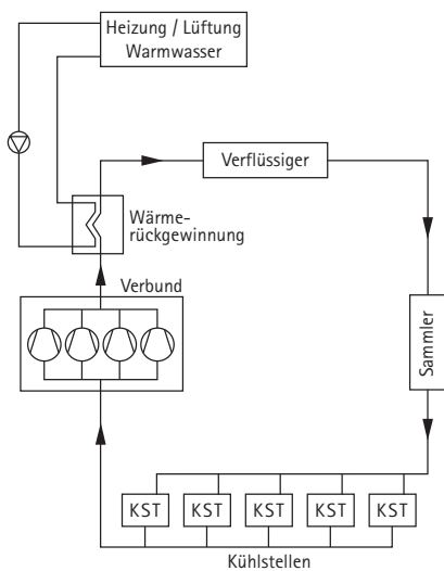
Verbundanlagenaufbau
